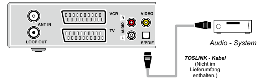
Receiver - Rückseite
