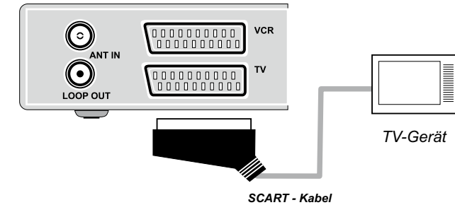
Receiver - Rückseite
