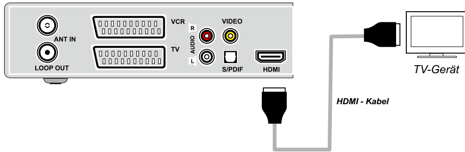
Receiver - Rückseite
