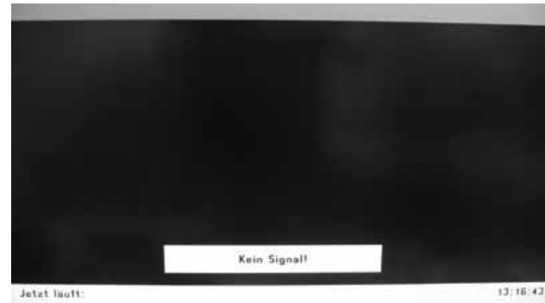
Kein Signal
